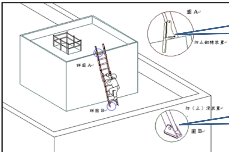
移動梯防止翻轉及滑溜裝置(一)
